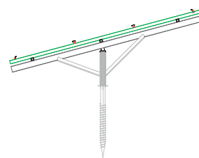
VISTA LATERAL
